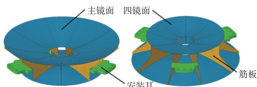
图 8 尺寸优化网格模型
