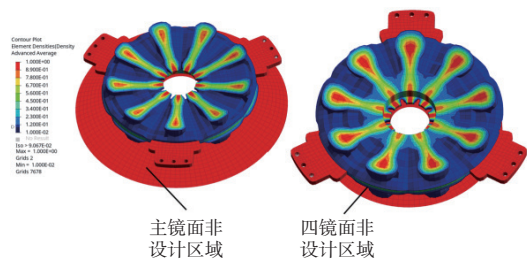
图6 拓扑材料密度分布图
