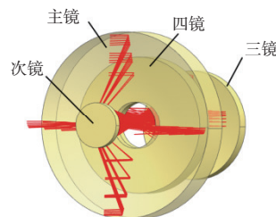
图4 同轴四反光路图
