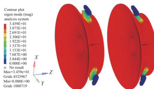
图 11 第一阶振型
