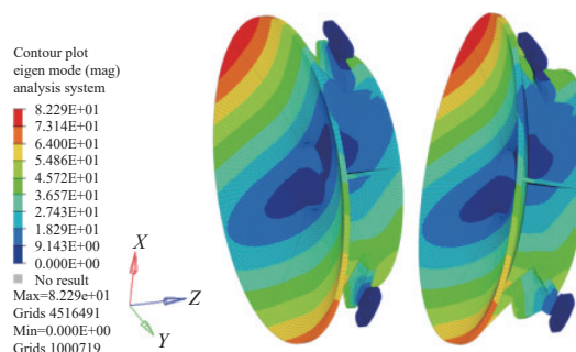
图 12 第二阶振型
