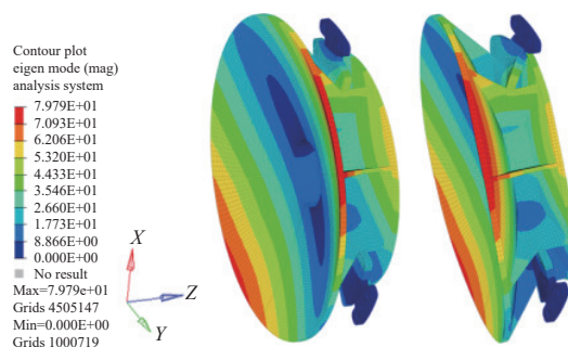
图 13 第三阶振型
