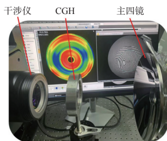
图 15 干涉仪检测面形测试过程
