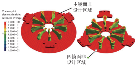
图7 材料密度大于0.6 kg/m 2 分布结果
