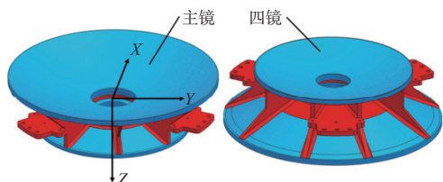
图 10 最终设计的主四镜模型
