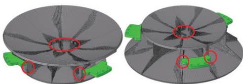
图 9 自由尺寸优化结果
