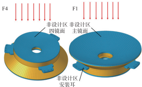
图5 拓扑优化有限元初始模型
